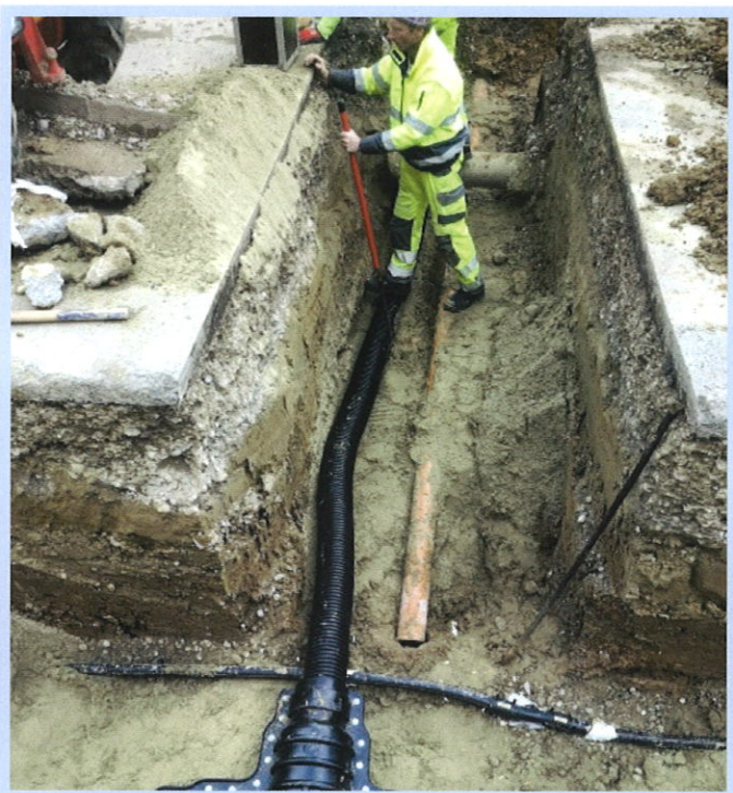
▲ Die Firma Wilhelm GmbH beauftragte den Bau einer Fernwärmeleitung in Unterrieden
